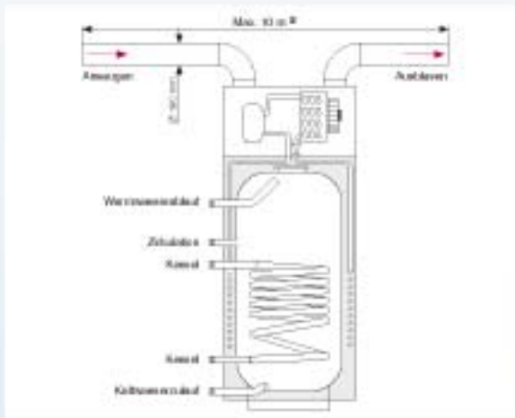
» Luft-Wasser-Wärmepumpe
